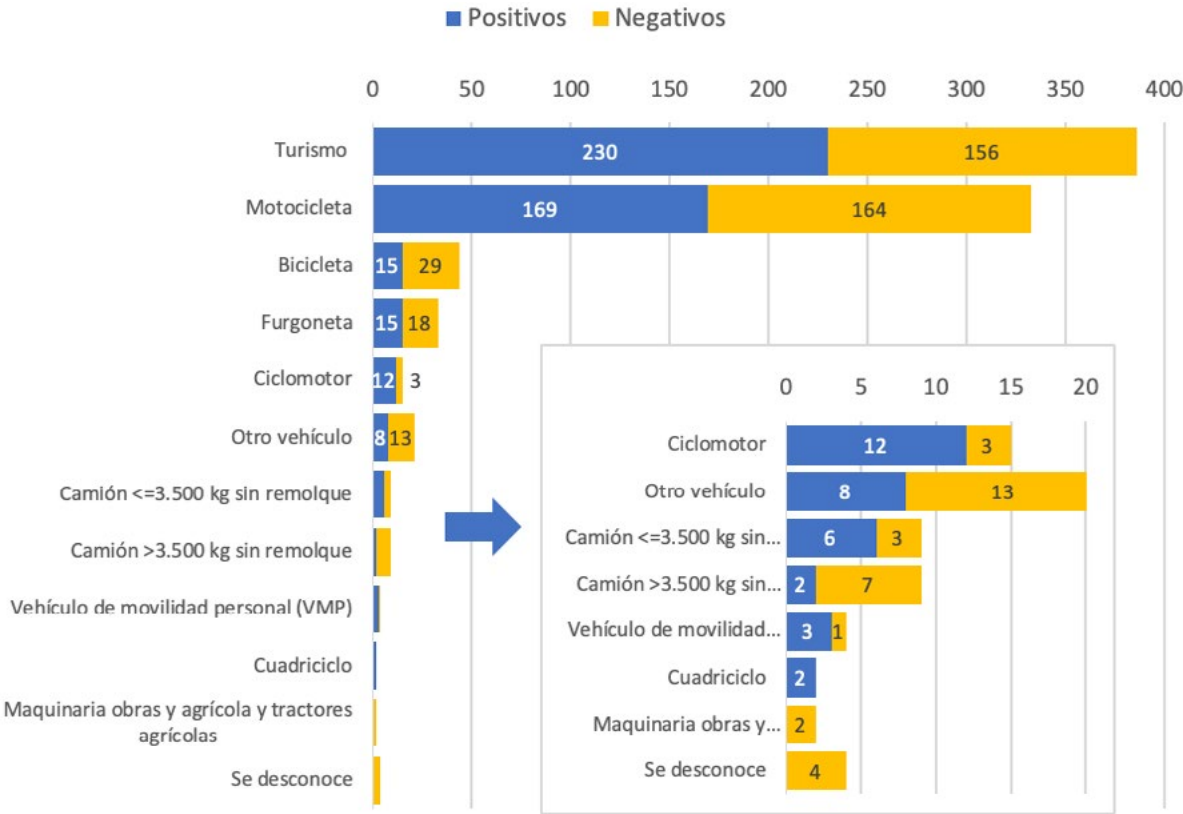
GRÁFICO 9: DISTRIBUCIÓN SEGÚN EL RESULTADO TOXICOLÓGICO Y EL TIPO DE VEHÍCULO (862 CONDUCTORES)
